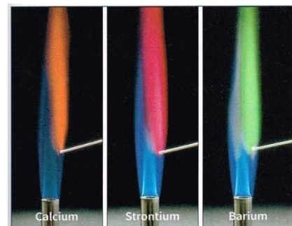
2. Flammenfärbung von Calcium, Strontium und Barium
